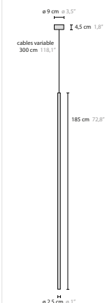
11040 H1 185
