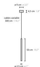
11005 H1 50
