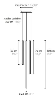
11050 H3
