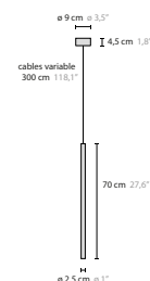
11010 H1 70
