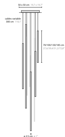
11052 H8
